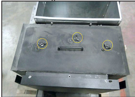
Ábra 7. A vízszintes füstnyílások a fedő lesterelése - 1
