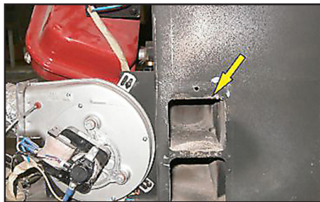
Ábra 10. A korom lepedék kitakarítása az ellenőrző nyílások keresztül a kandalló két oldalán - 1. lépés (modell 25kW)
