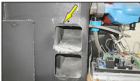
Ábra 10. A korom lepedék kitakarítása az ellenőrző nyílások keresztül a kandalló két oldalán - 2. lépés (modell 18 Kw-25kW)
