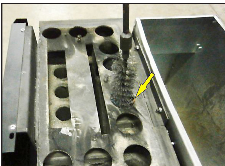
Ábra 9. A kialakult korom lepedék kitakarítása drótkéfével
