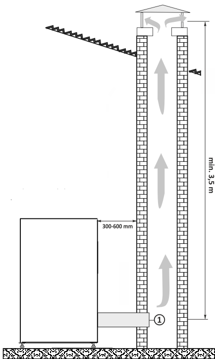
2. Ábra A pelletkandalló csatlakozása a kéményhez
